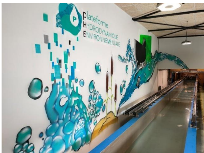
Canal hydrodynamique de la plateforme hydrodynamique environnementale (pHE) de l'Institut Pprime, CNRS-Université de Poitiers Mesure PIV de l'écoulement en interaction fluide structure sur une ligne de maquettes calibrées de tiges flexibles.
