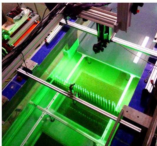
Canal hydrodynamique de la plateforme hydrodynamique environnementale (pHE) de l'Institut Pprime, CNRS-Université de Poitiers Mesure PIV de l'écoulement en interaction fluide structure sur une ligne de maquettes calibrées de tiges flexibles.
